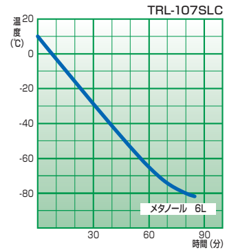
冷却能力表 TRL-107SL/TRL-107SLC
