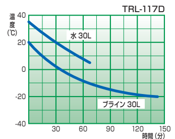
冷却能力表 TRL-117D
