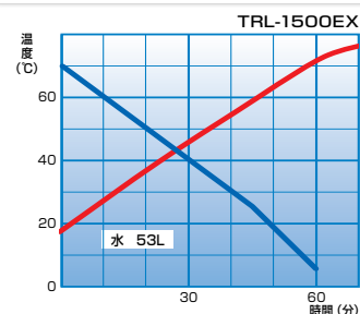
TRL-1500EX 冷却能力
