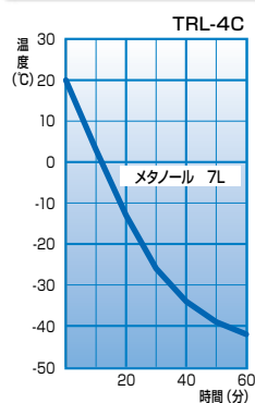
冷却能力表 TRL-4C
