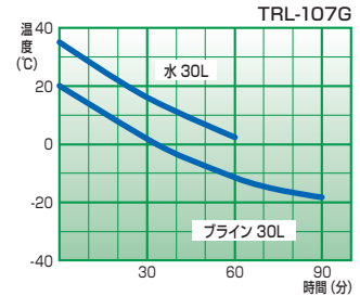
冷却能力表 TRL-107G
